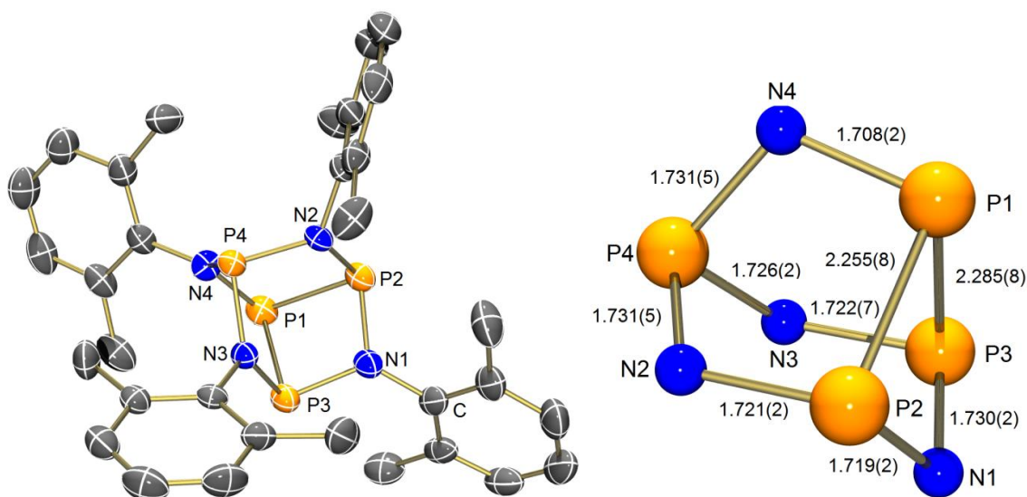
Abbildung 19. Links: ORTEP-Darstellung von 11 im Kristall (H-Atome nicht dargestellt). Die thermischen Ellipsoide entsprechen 50 % Aufenthaltswahrscheinlichkeit bei 173 K. Rechts: Darstellung der P_4N_4 -Einheit mit Abständen in Å. Ausgewählte Bindungswinkel [°]: P2–P1–P3 75.72(3), N4–P1–P3 96.54(8), N1–P2–P1 83.34(7), N2–P2–P1 93.18(7), N3–P3–N1 105.85(9), N3–P3–P1 92.68(7), N1–P3–P1 82.19(8), N3–P4–N4 96.64(10), N3–P4–N2 99.24(9), N4–P4–N2 96.27(9), P2–N1–P3 107.86(11), P2–N2–P4 118.71(10), P3–N3–P4 119.02(11) P1–N4–P4 111.83(11).
