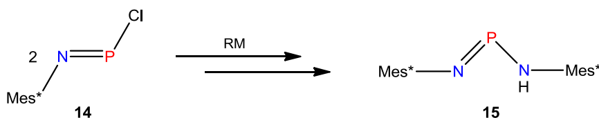
Schema 21. Reduktion des monomeren \text{Mes}^*-\text{N}=\text{P}-\text{Cl} zum Iminoaminophosphan (RM = Mg, Li, \text{Cp}_2\text{Ti}(\text{btmsa}) und [\text{Cp}_2\text{TiCl}]_2 ).
