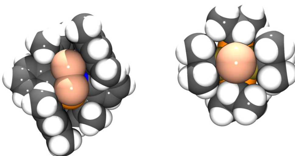
Abbildung 26. Kalottenmodell von 18 (links) und t\text{-BuB}(\mu\text{-Se})(\mu\text{-P}^i\text{Pr}_2)_2\text{B}^i\text{Bu} (rechts).
