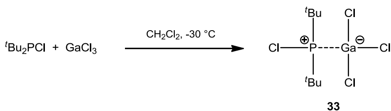
Schema 37. Reaktion von {}^t\text{Bu}_2\text{P}(\text{Cl}) mit \text{GaCl}_3 .
