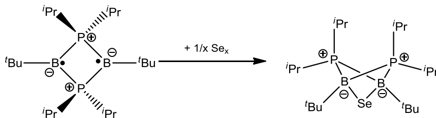
Schema 26. Darstellung des Selenderivats nach Bertrand. [93]
