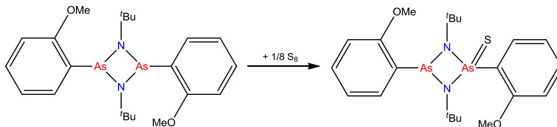
Schema 23. Einzige bekannte Oxidation eines schwereren cyclo -Dipnicta(III)diazans mit einem Chalkogen. [86]
