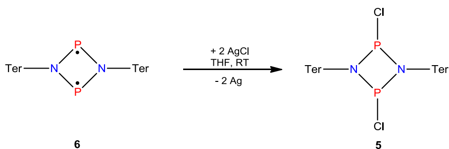
Schema 33. Reaktion von 6 mit AgCl.
