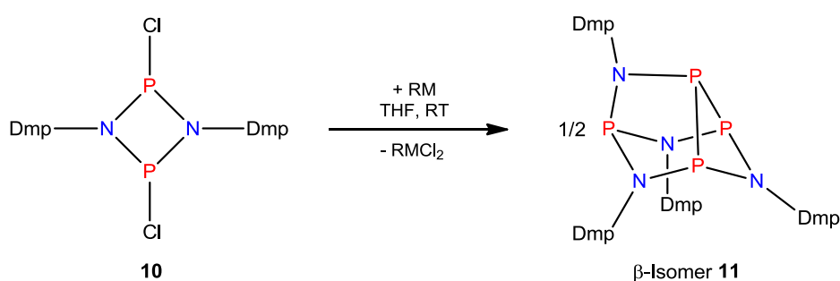
Schema 19. Reduktion von 10 mit \text{Cp}_2\text{Ti}(\text{btmsa}) oder Magnesium.
