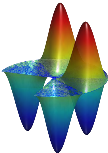
Eigenfunktion des Laplaceoperators auf einem Dreiviertelkreis
